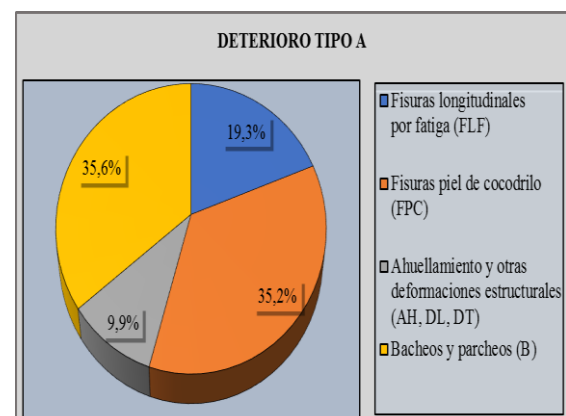
Figura 5 Deterioros de tipo A registrados en el tramo de estudio.
