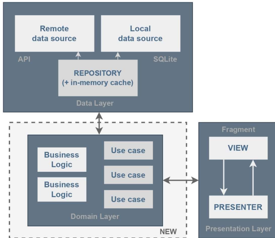
Figura 2. Estructura de la implementación de arquitectura limpia aplicaciones Android. Fuente: [17].
