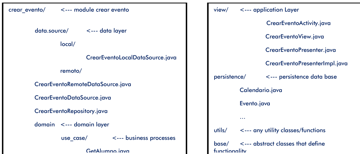
Figura 5. Estructura de carpetas de uno de los módulos del aplicativo móvil del Educar Teacher basado en arquitectura limpia. Fuente: elaboración propia.
