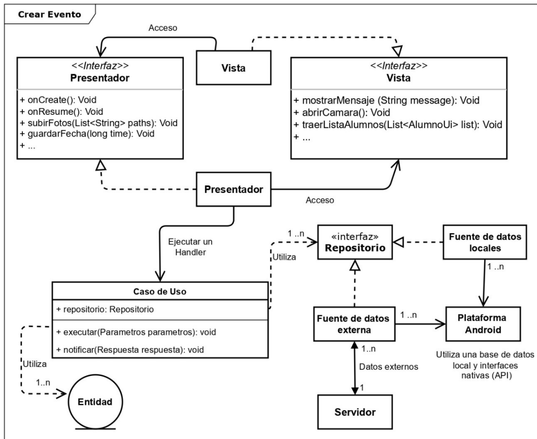
Figura 4. Diagrama de flujo de uno de los módulos del aplicativo móvil Educar Teacher basado en arquitectura limpia. Fuente: elaboración propia.
