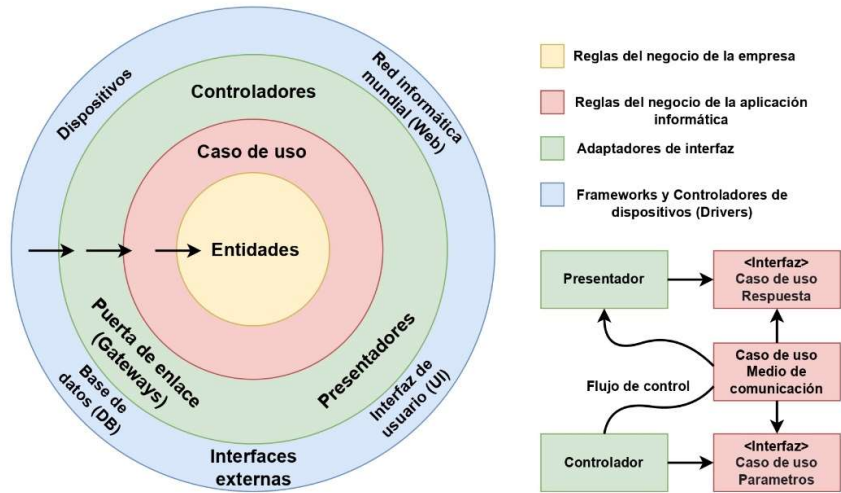
Figura 3. La regla de la dependencia de arquitectura limpia. Fuente: [16].
