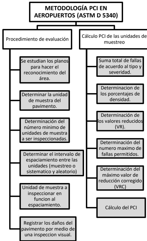
Fig. 4. Flujograma PCI en Aeropuertos (ASTM D 5340)
