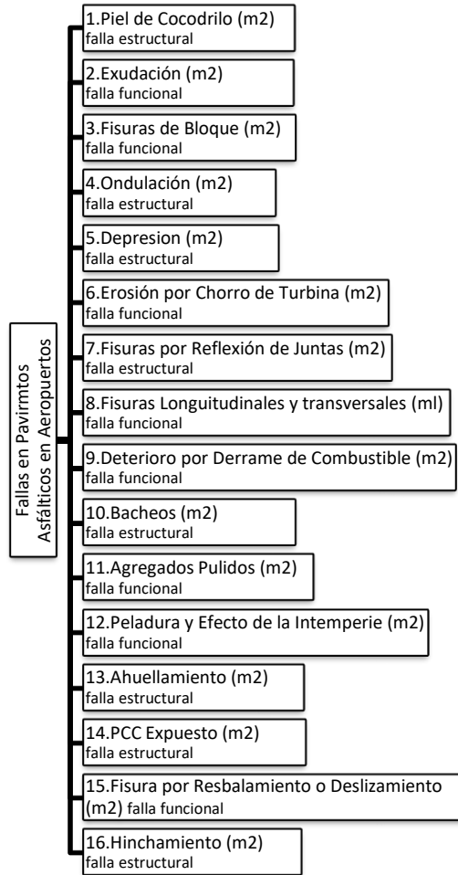
Fig. 2. Diagrama de fallas en pavimentos asfálticos en Aeropuertos (ASTM D 5340)
