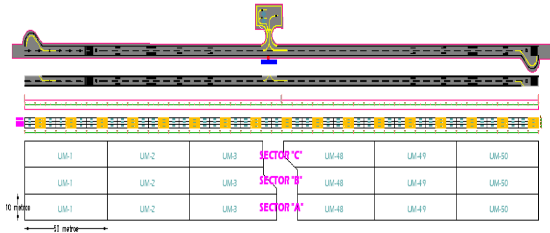
Fig. 3. Lado aire del aeropuerto de Huánuco Perú con su señalización, progresiva y unidades de muestra a estudiar (Propia).
