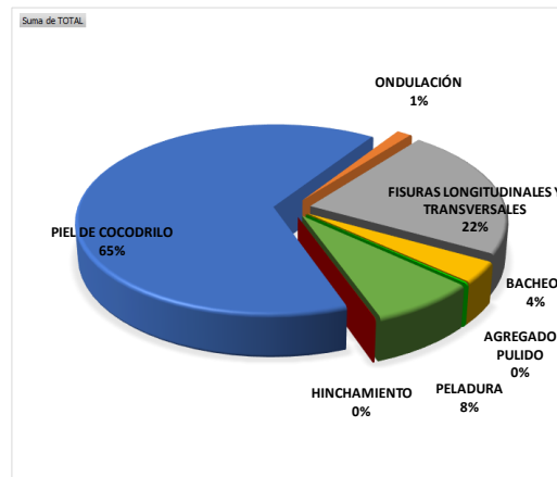
Fig. 5. Fallas encontradas en la pista de aterrizaje del aeropuerto de Huánuco.
