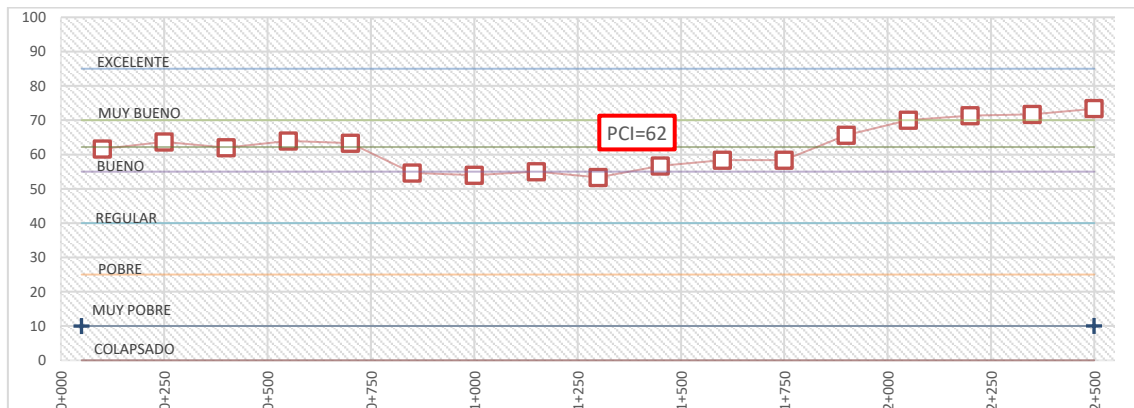
Fig. 6. Grafica del índice de condición de pavimento (PCI) de la pista de aterrizaje del aeropuerto Huánuco.
