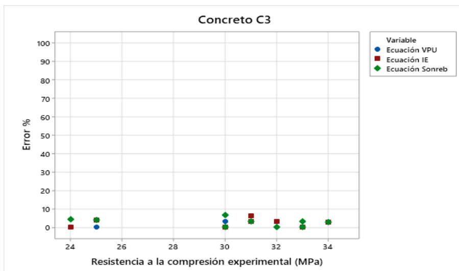
Figura 16. Estimación de f'c a partir del porcentaje de error de ecuaciones analíticas para concreto con adición fibra de polipropileno 0,21 %. Fuente: el autor
