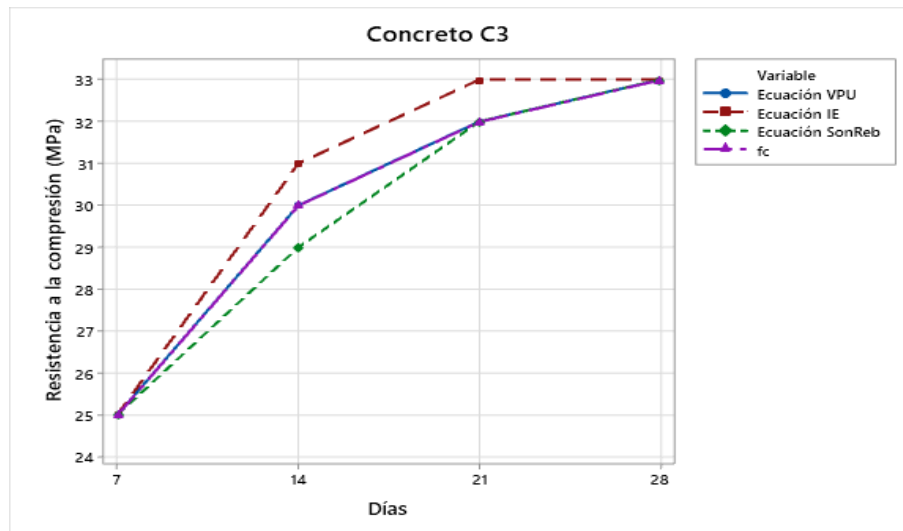
Figura 13. Análisis de la f'c mediante modelos de ecuaciones para concreto con adición de fibra de polipropileno 0,21%. Fuente: el autor
