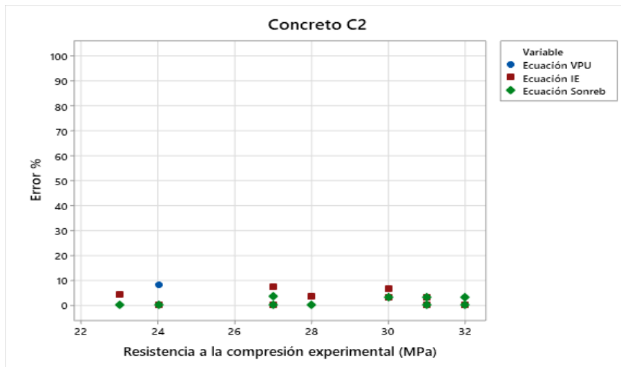
Figura 15. Estimación de f'c a partir del porcentaje de error de ecuaciones analíticas para concreto con adición fibra de acero 5 %. Fuente: el autor
