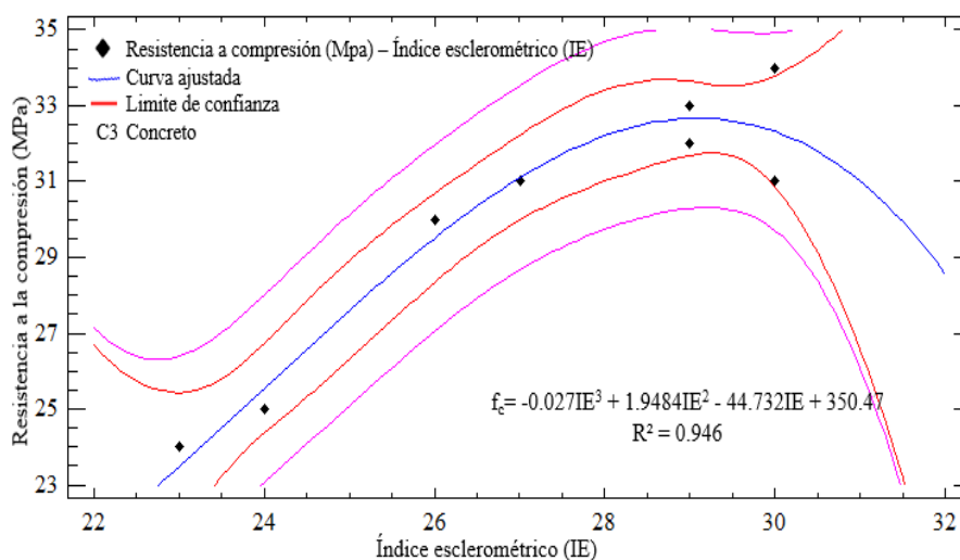
Figura 11. Curvas de correlación entre f_c e IE del concreto con fibra de polipropileno 0,21 %. Fuente: el autor
