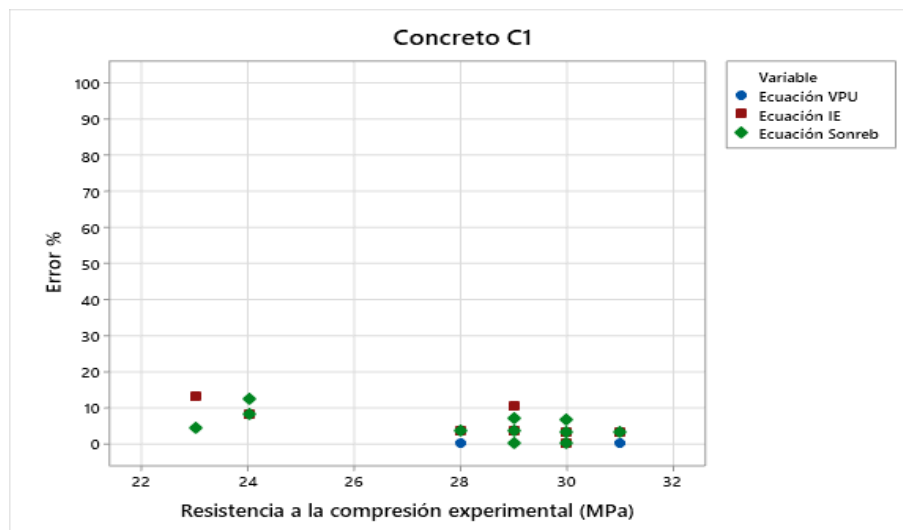
Figura 14. Estimación de f'c a partir del porcentaje de error de ecuaciones analíticas para concreto convencional. Fuente: el autor
