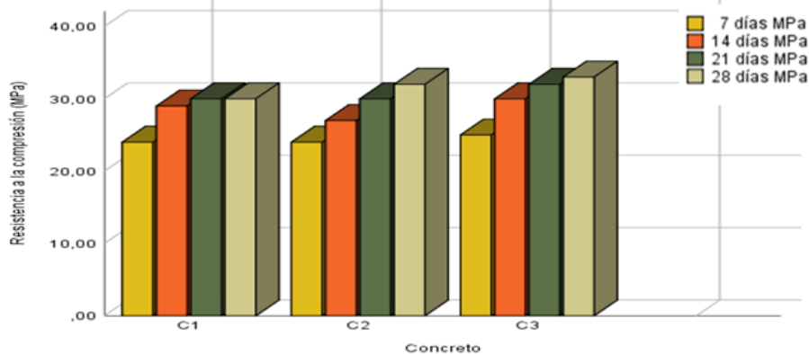
Figura 3. Resistencia a la compresión. Fuente: el autor
