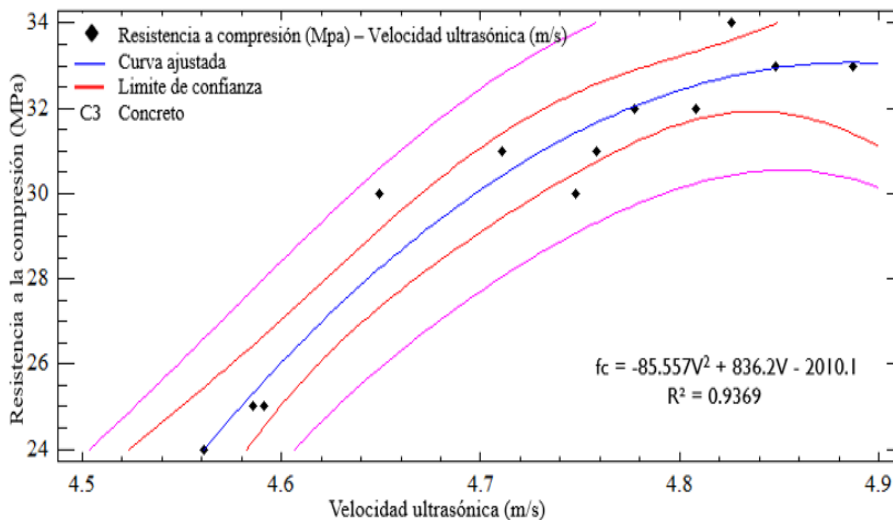
Figura 8. Curvas de correlación entre f_c y VPU del concreto con polipropileno 0,21 %. Fuente: el autor
