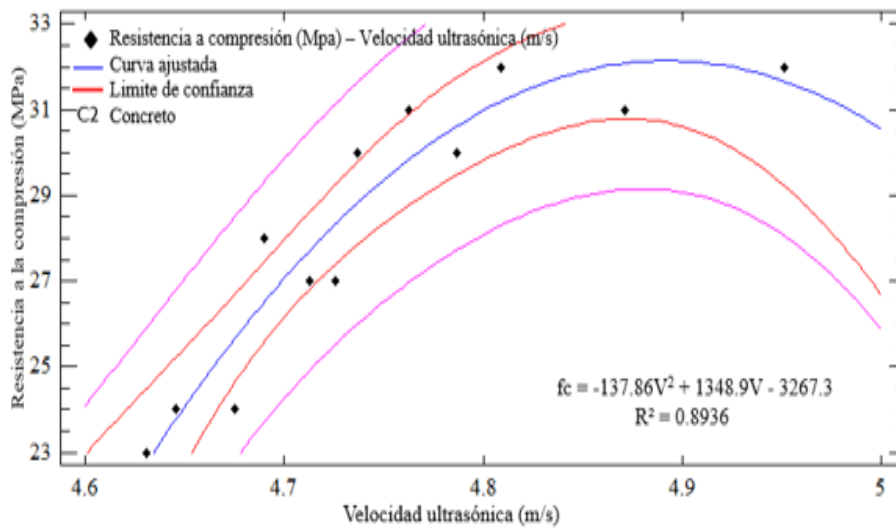
Figura 7. Curvas de correlación entre f_c y VPU del concreto con fibra de acero 5 %. Fuente: el autor
