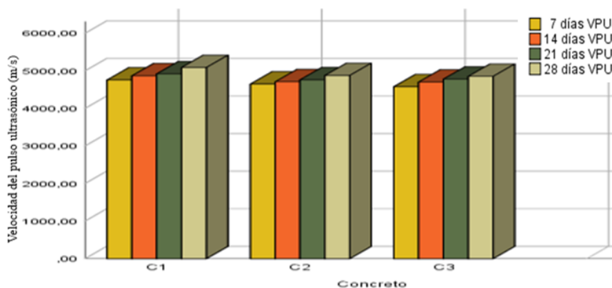
Figura 4. Velocidad del pulso ultrasónico. Fuente: el autor
