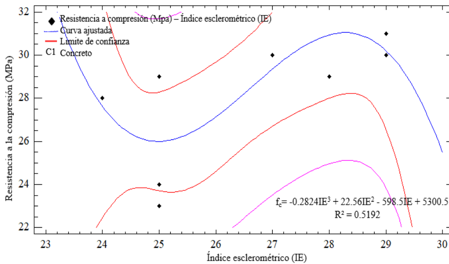
Figura 9. Curvas de correlación entre f'_c e IE del concreto convencional. Fuente: el autor
