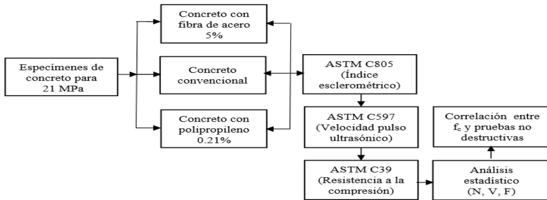
Figura 1. Diagrama de flujo para el cálculo analítico de la resistencia del concreto. Fuente: el autor
