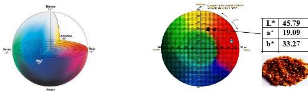
Figura 7 Espacio CIELab
