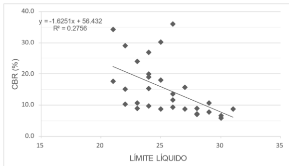
Figura 4. CBR vs límite líquido Fuente: Elaboración propia
