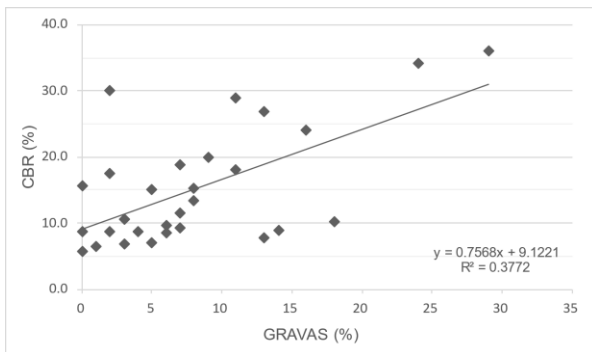
5 Figura 1. CBR vs Gravas (%)
