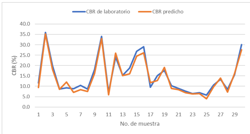
Figura 8. Comparación entre CBR de laboratorio y CBR predicho por la ecuación de correlación con el mejor nivel de ajuste. Fuente: Elaboración propia
