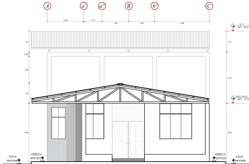
ELEVACION FRONTAL ESCALA 1/50
