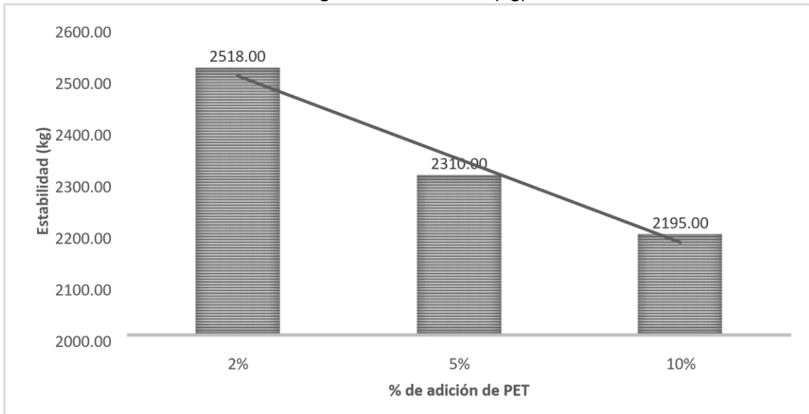
Figura 6. Estabilidad (kg)
