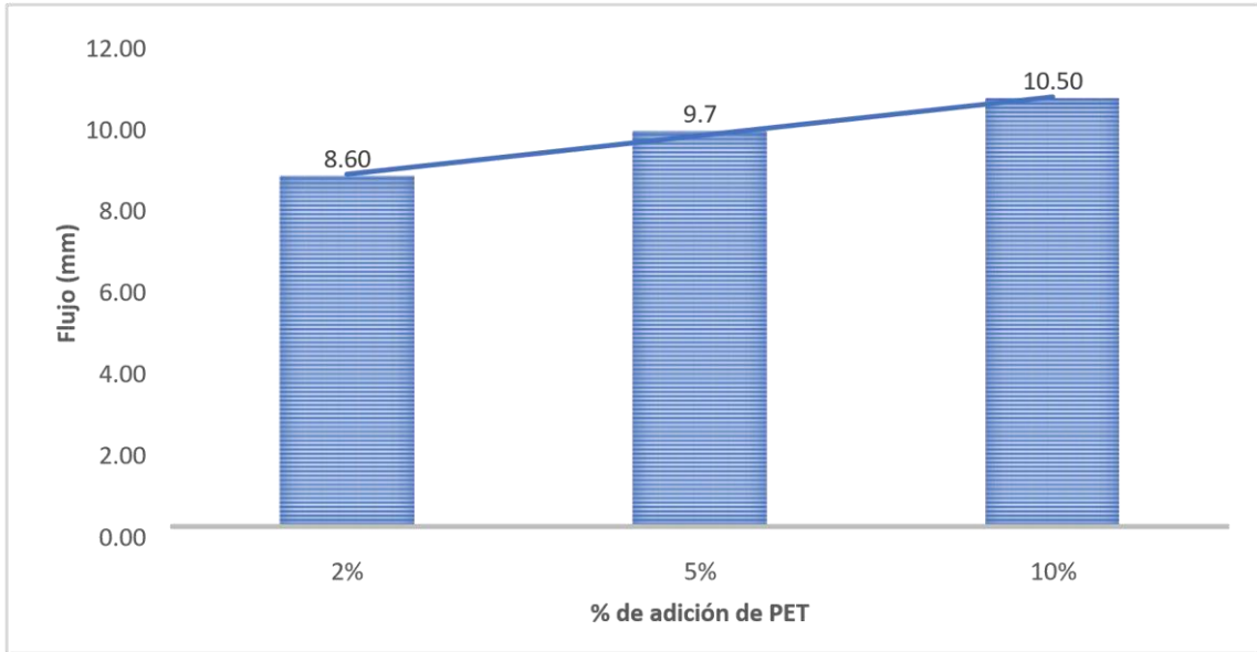
Figura 5. Flujo (mm)
