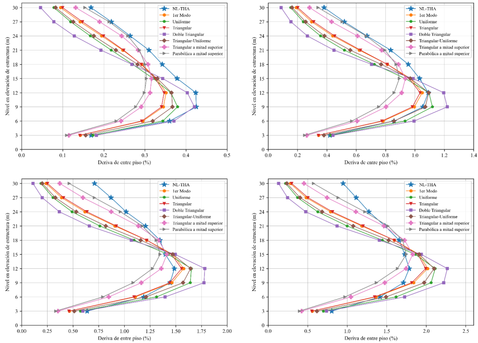
Figura 13 Derivas de entre piso para intensidad leve (superior-izquierda), moderada (superior-derecha), severa (inferior-izquierda) y crítica (inferior-derecha) de la estructura de 10 niveles.
