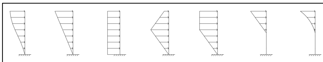
Figura 3 Patrones de distribución de carga. Fuente: Elaboración propia.
