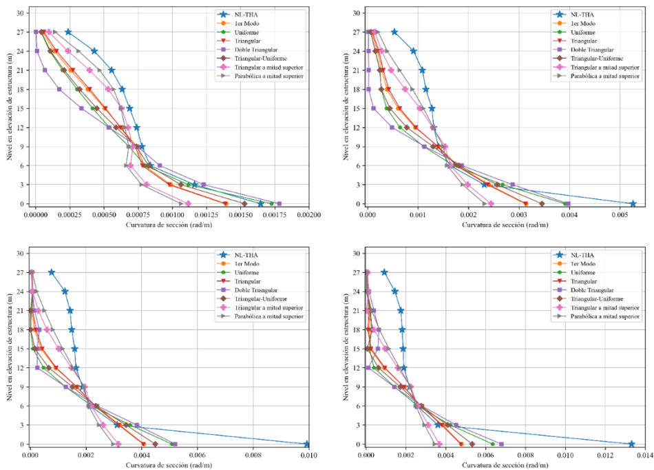
Figura 14 Curvatura de sección en la base de las columnas centrales para intensidad leve (superior-izquierda), moderada (superior-derecha), severa (inferior-izquierda) y crítica (inferior-derecha) de la estructura de 10 nivel
