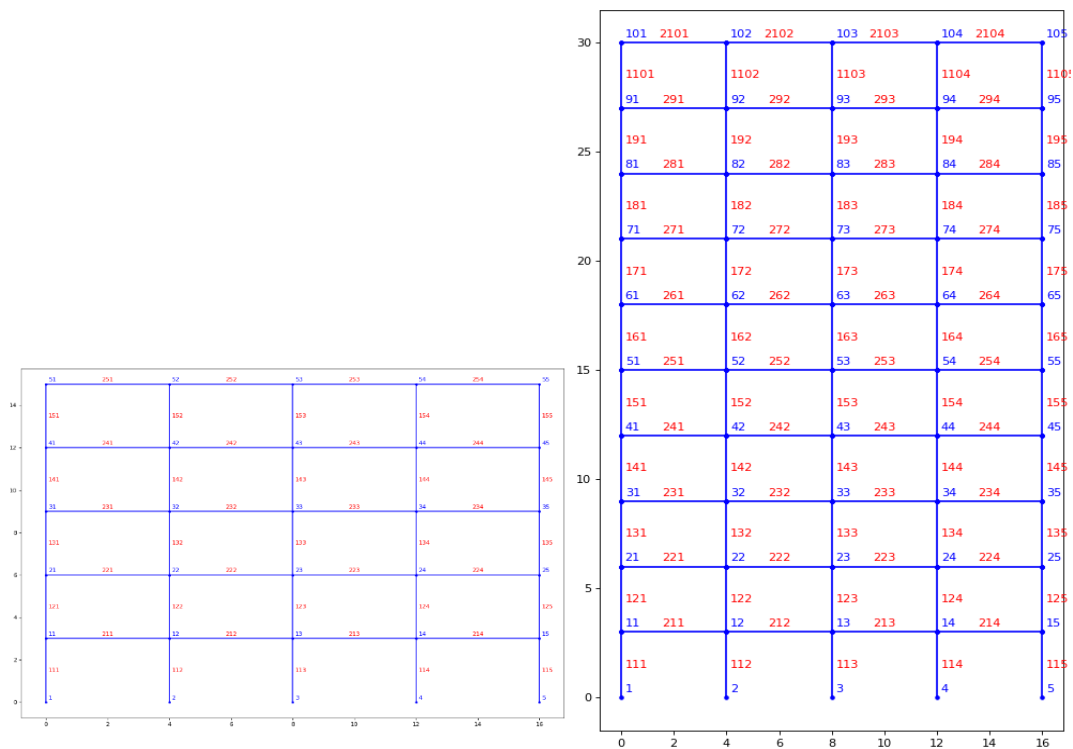
Figura 5 Modelos estructurales en dos dimensiones construidos en OpenSees. Estructura de 5 niveles (izquierda), estructura de 10 niveles (derecha). Fuente: Elaborada y extraída de OpenSeesPy.
