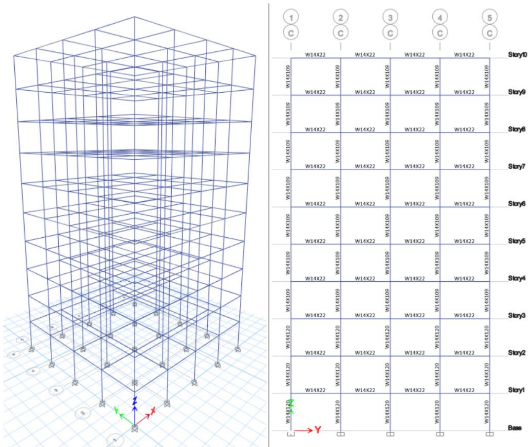
Figura 2 Vista en 3D de estructura propuesta (10 niveles) y vista en elevación del pórtico elegido (C) para el análisis de las estructuras. Fuente: Elaborada y extraída de ETABS.
