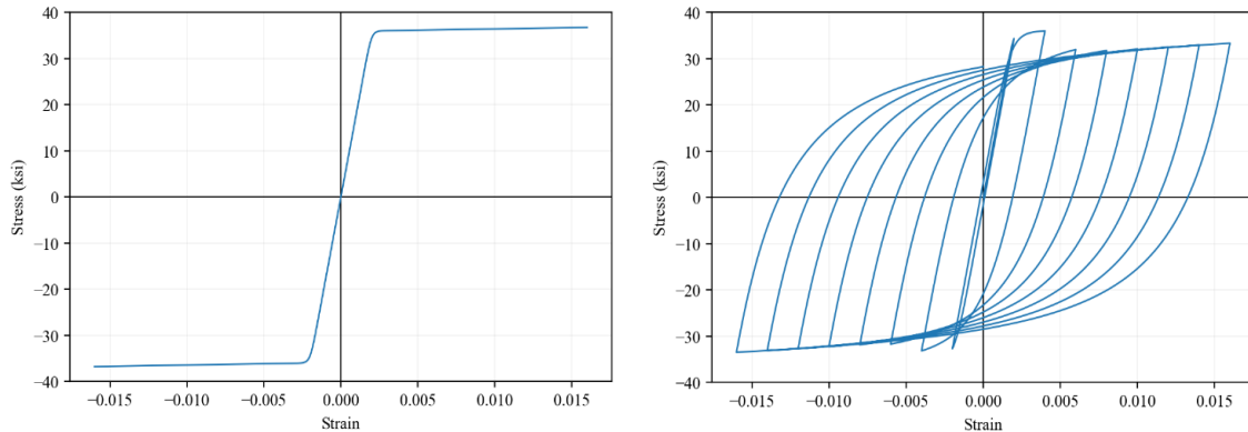
Figura 7 Modelo de acero estructural ASTM A36; comportamiento monotónico (izquierda), comportamiento histérico (derecha) Fuente: Elaborada y extraída de OpenSeesPy.
