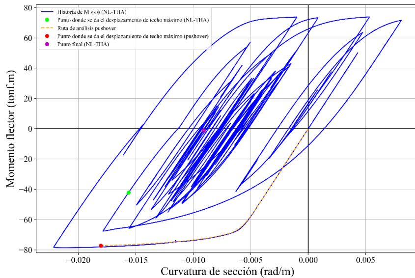
Figura 16 Gráfica de Momento-Curvatura obtenidas de diferentes análisis empleando la señal Ica 2007 escalada a intensidad crítico (PGA = 0.95g).
