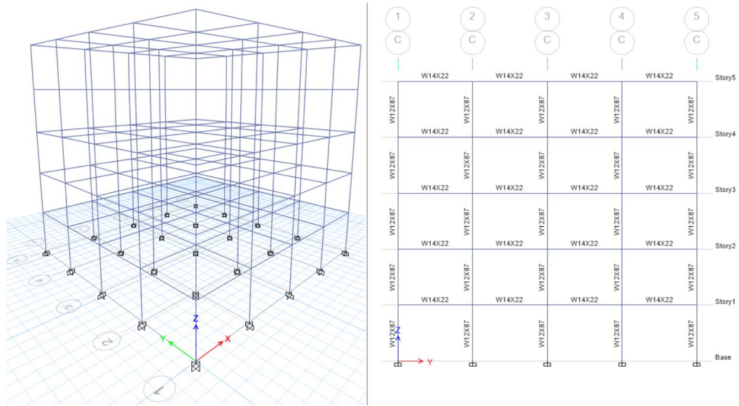
Figura 1 Vista en 3D de estructura propuesta (5 niveles) y vista en elevación del pórtico elegido (C) para el análisis de las estructuras. Fuente: Elaborada y extraída de ETABS.
