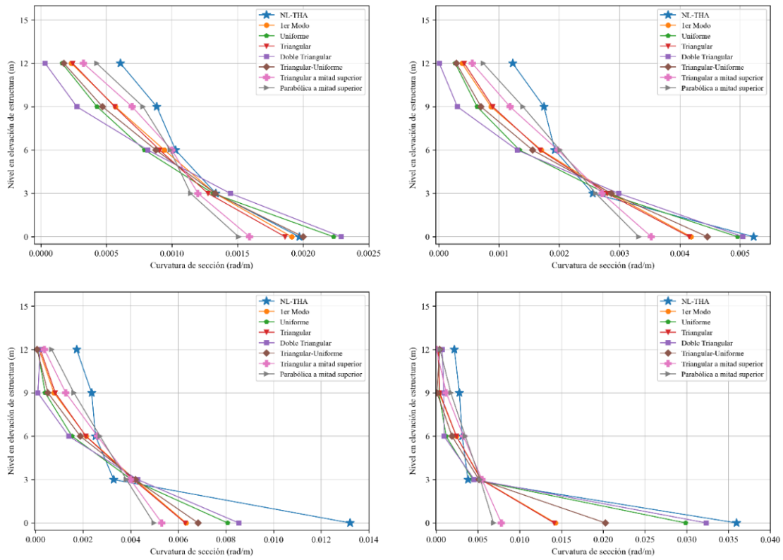
Figura 10 Curvatura de sección en la base de las columnas centrales para intensidad leve (superior-izquierda), moderada (superior-derecha), severa (inferior-izquierda) y crítica (inferior-derecha) de la estructura de 5 niveles.
