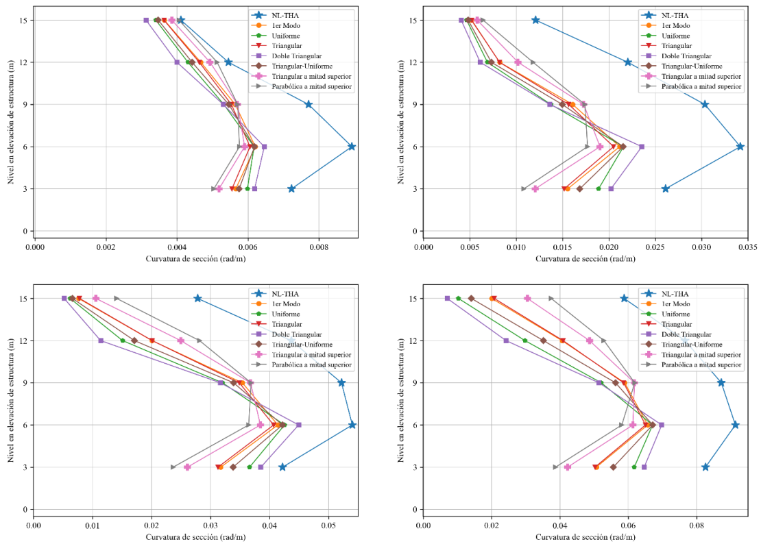
Figura 11 Curvatura de sección en las vigas centrales para intensidad leve (superior-izquierda), moderada (superior-derecha), severa (inferior-izquierda) y crítica (inferior-derecha) de la estructura de 5 niveles.
