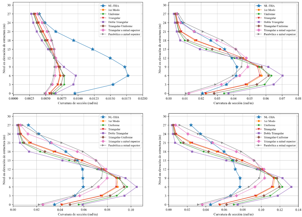
Figura 15 Curvatura de sección en las vigas centrales para intensidad leve (superior-derecha), moderada (superior-derecha), severa (inferior-izquierda) y crítica (inferior-derecha) de la estructura de 10 niveles.
