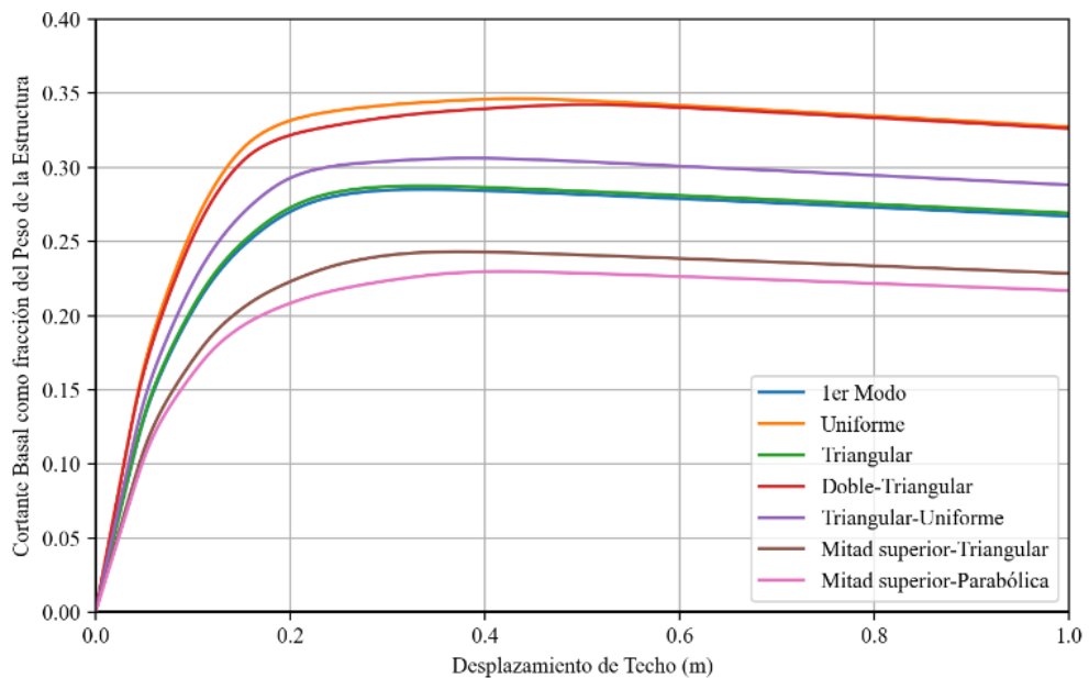
Figura 8 Curvas de capacidad para diferentes patrones de distribución de carga para la estructura de 5 niveles.
