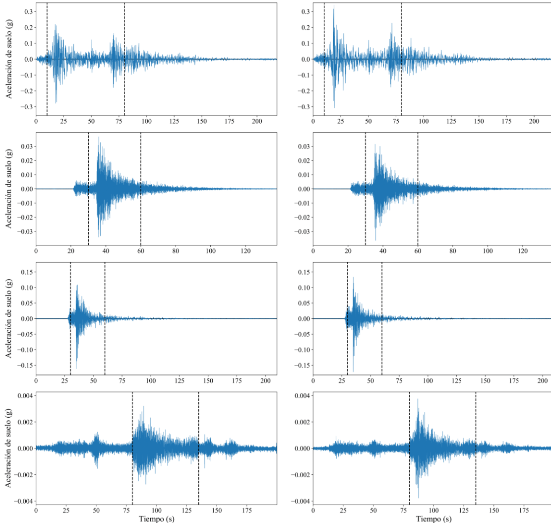
Figura 4 Registros de aceleraciones de los sismos Ica 2007, Lima 2018, Piura 2021 y Tacna 2022 (de arriba hacia abajo). Fuente: Elaborada propia.
