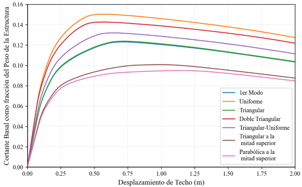
Figura 12 Curvas de capacidad para diferentes patrones de distribución de carga para la estructura de 10 niveles.
