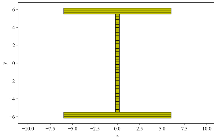
Figura 6 Sección de fibras para elementos basados en fuerza. Fuente: Elaborada y extraída de OpenSeesPy.
