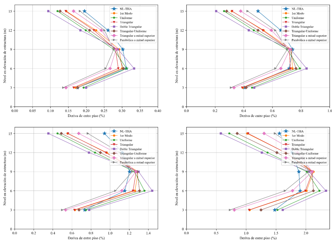
Figura 9 Derivas de entre piso para intensidad leve (superior-izquierda), moderada (superior-derecha), severa (inferior-izquierda) y crítica (inferior-derecha) de la estructura de 5 niveles.
