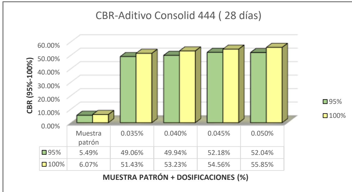
Figura 2. CBR del suelo mejorado con aditivo Consolid 444. Fuente: los autores
