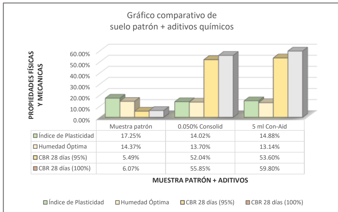
Figura 4. Gráfico comparativo de aditivos químicos. Fuente: los autores
