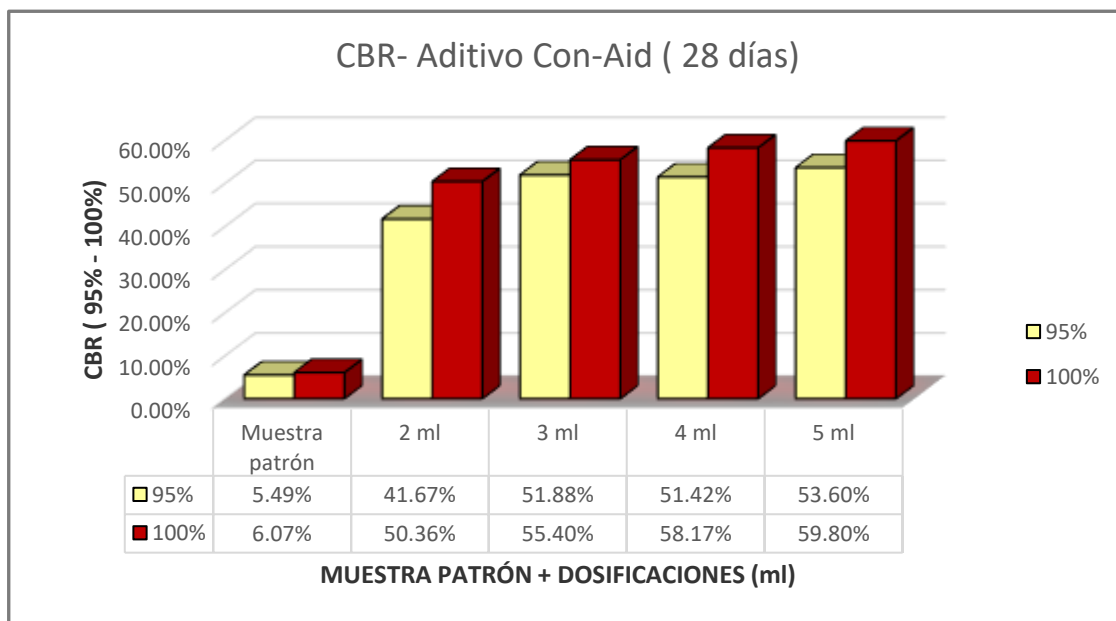
Figura 3. CBR del suelo mejorado con aditivo Con-Aid. Fuente: los autores
