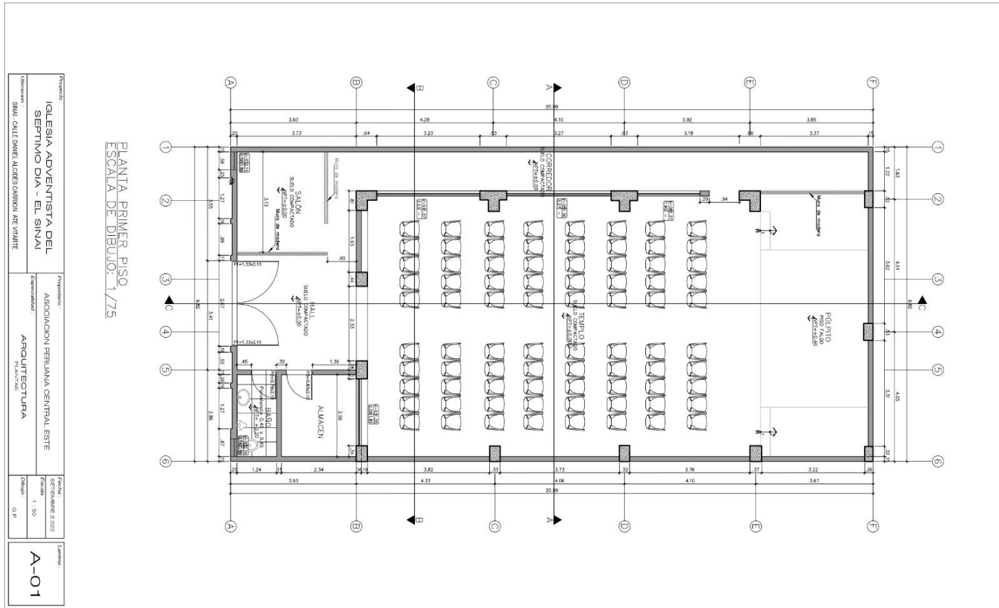
Figura 5. Plano de una iglesia adventista representativa
